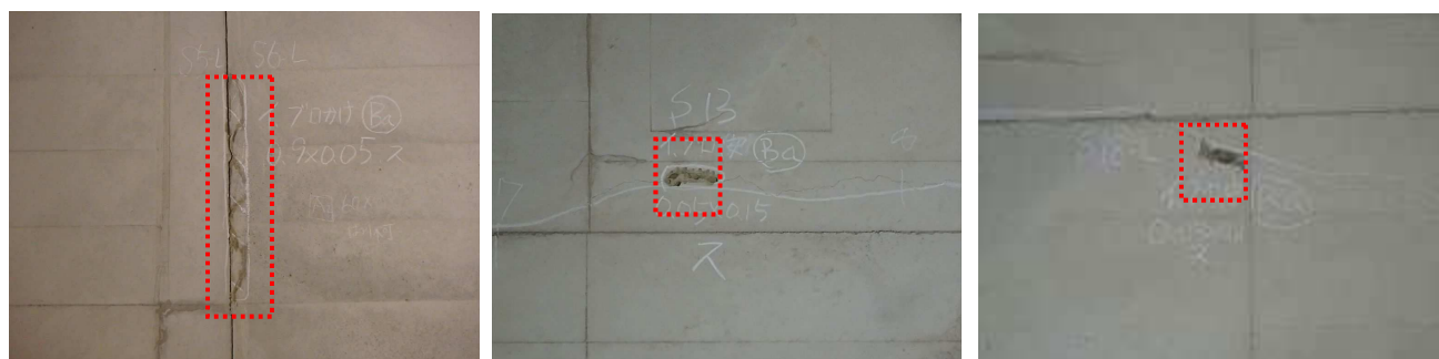
写真5.1 Ⅲ判定変状箇所（左からS006、S013、S018）
